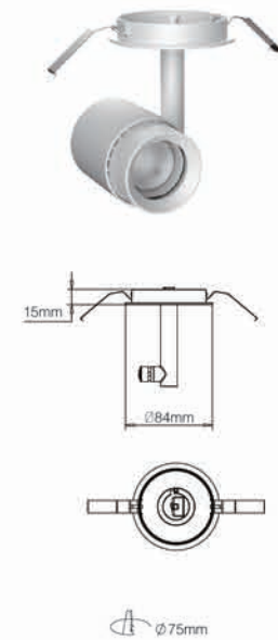
万向头
