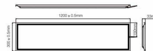
集成吊顶
