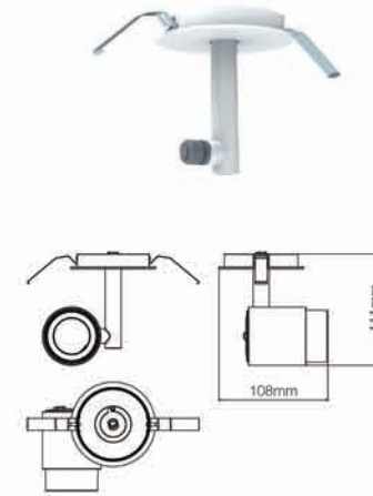
万向头
